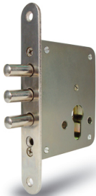
Фиг. 1101.23-24 – механизъм с палец и ръкохватка, с диаметър на цилиндъра 15 mm. 1101.21 – с диаметър на цилиндъра 15 mm. 1101.22 – с диаметър на цилиндъра 15 mm. 1101.23 – с диаметър на цилиндъра 15 mm. 1101.24 – с диаметър на цилиндъра 15 mm.
